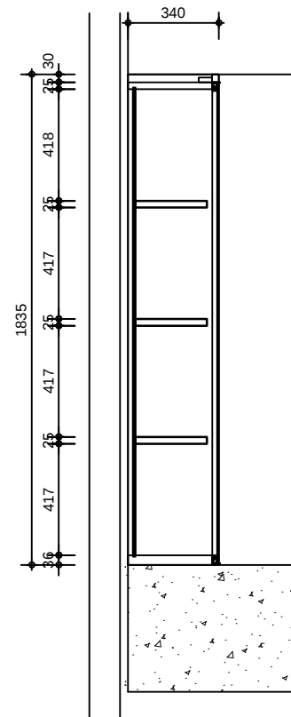
E-E剖面图
