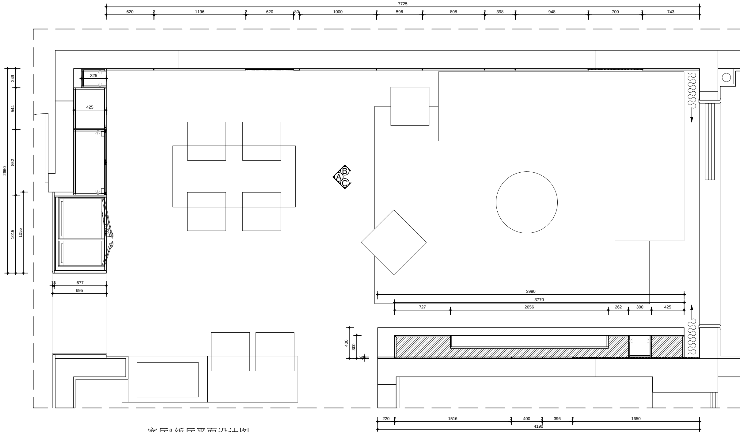
客厅&饭厅平面设计图
