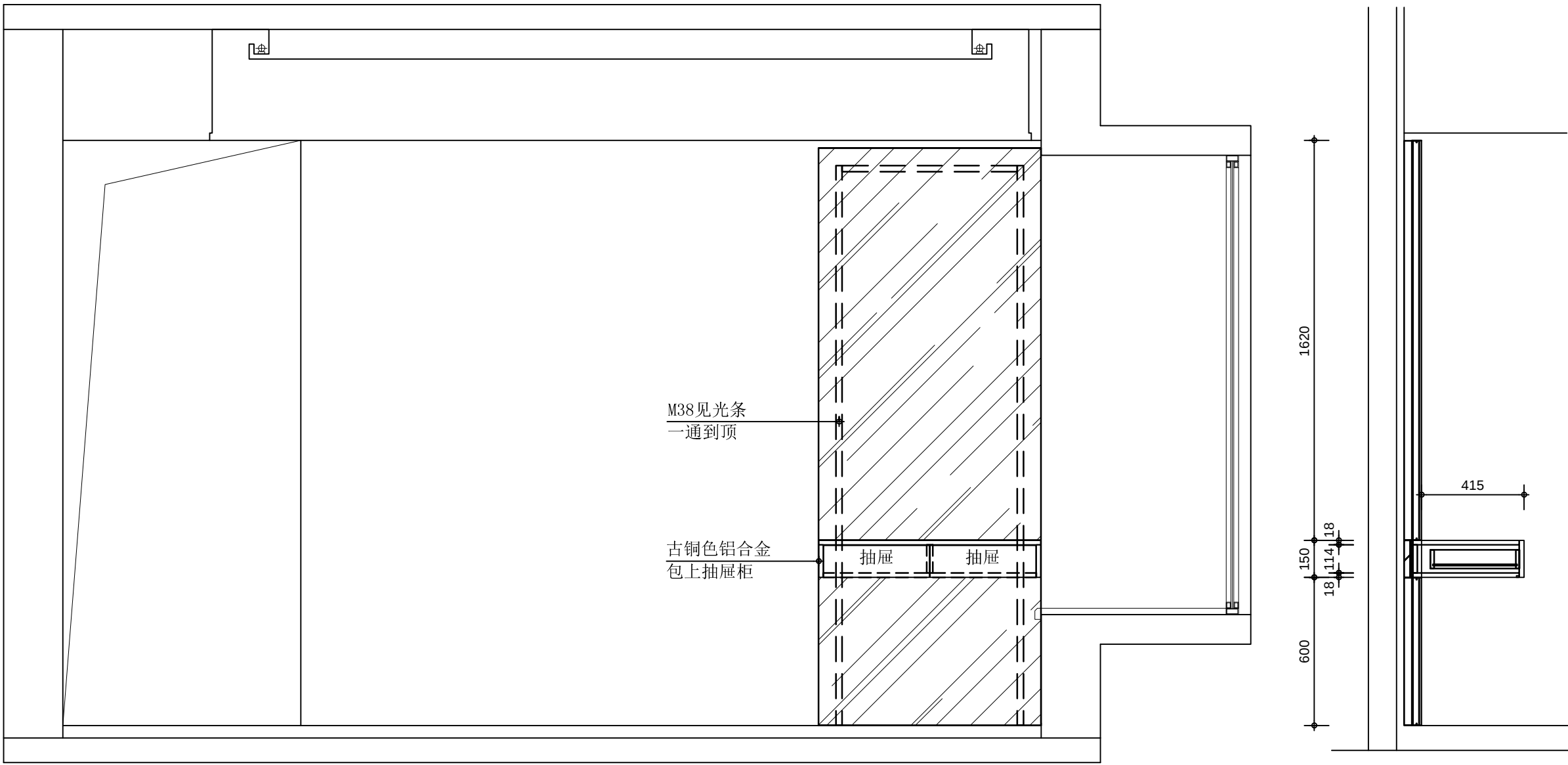
ELEVATION C 外观图
