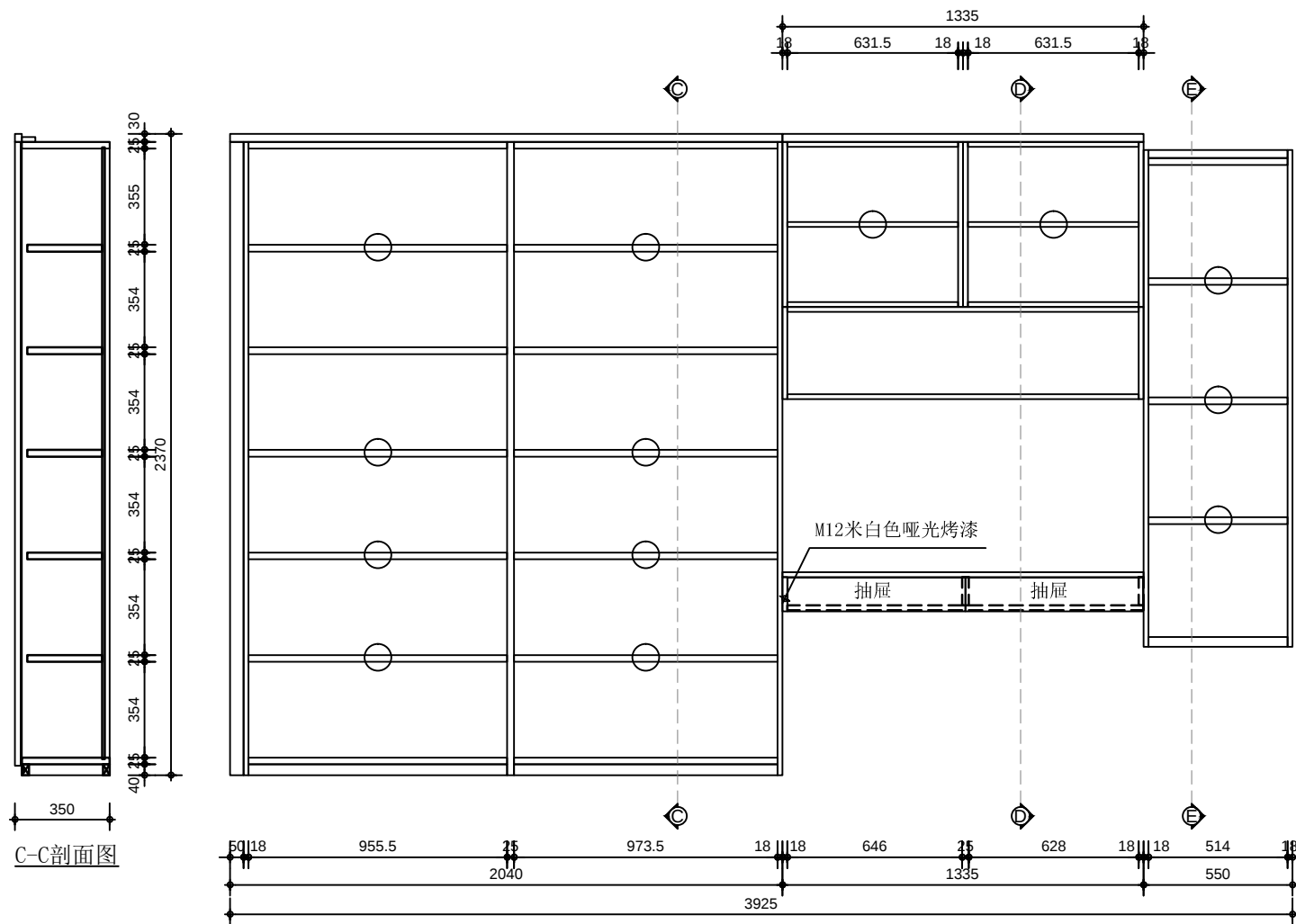
ELEVATION C 内部结构图
