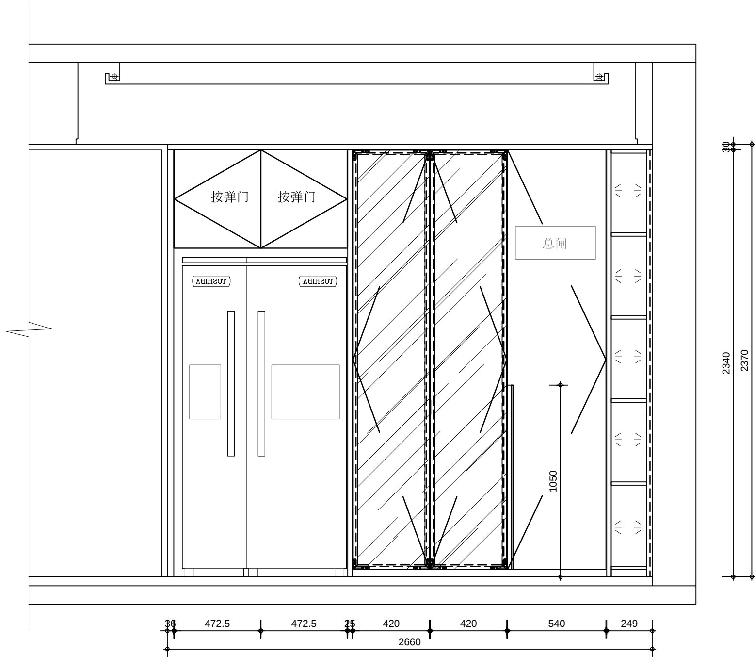
ELEVATION A 外观图
