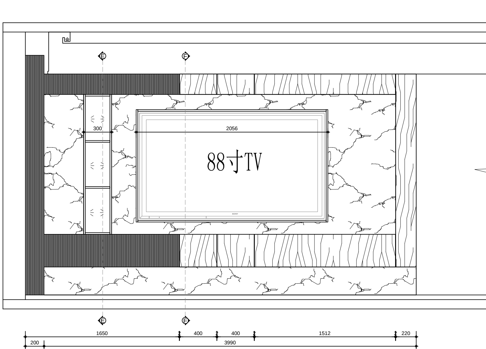
ELEVATION C 外观图
