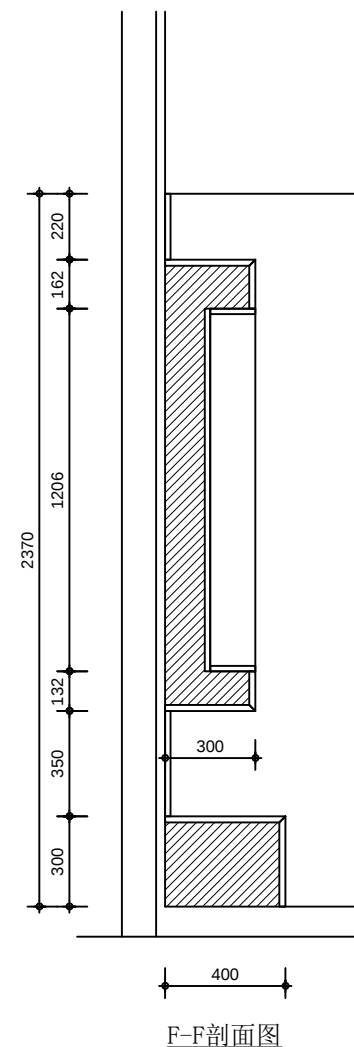
F-F剖面图
