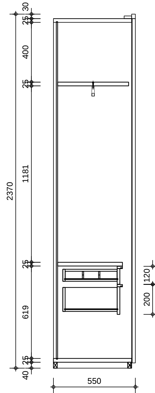
B-B剖面图
