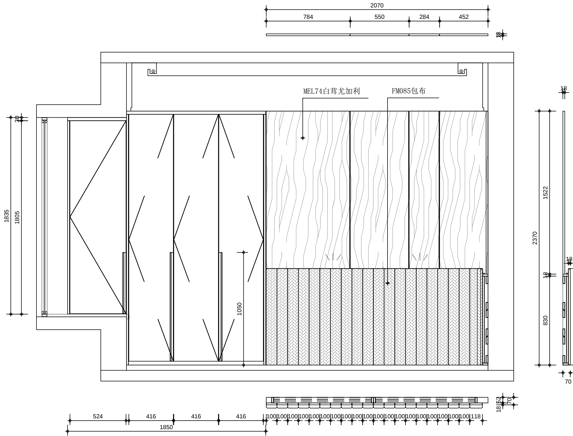
ELEVATION A 外观图
