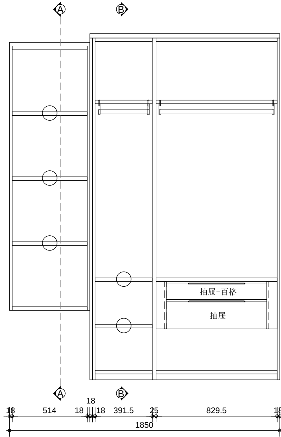
ELEVATION A 内部结构图
