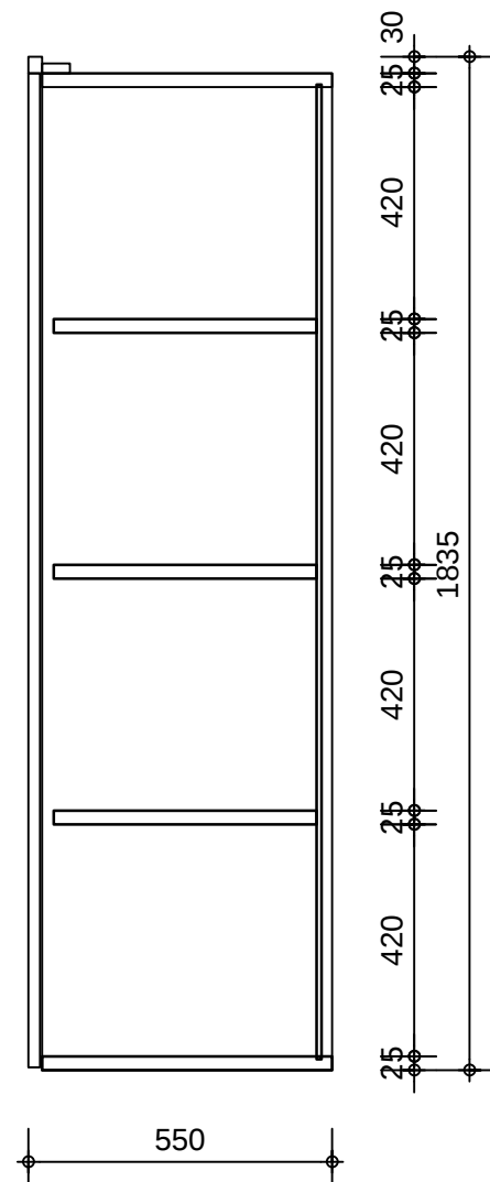
A-A剖面图
