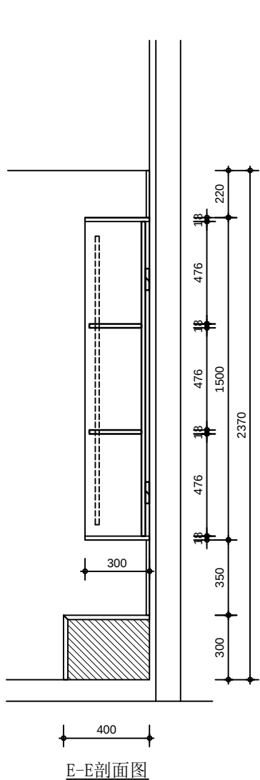
E-E剖面图
